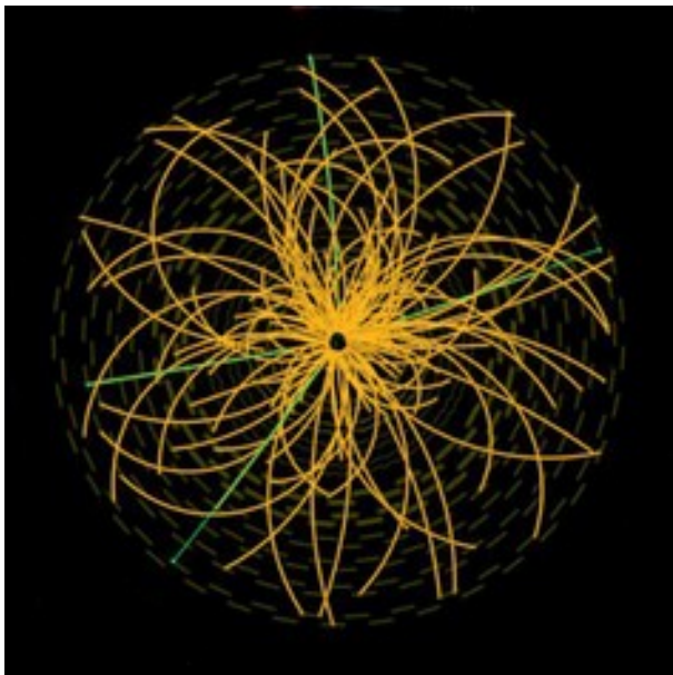
Бозон Хиггса - названный физиками «частицей Бога»
